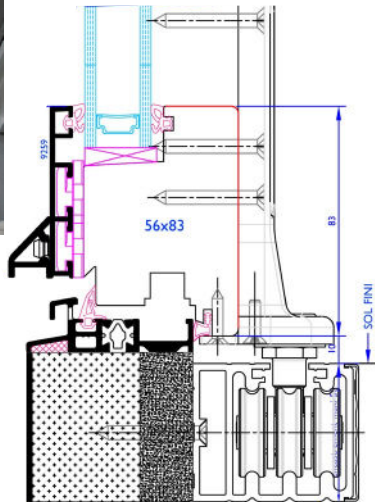
passage aisé - seuil encastré (20mm) - (PMR)
