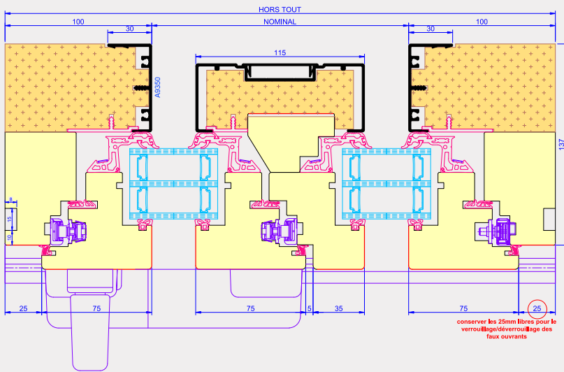
Coupe horizontale (Dormant et ouvrant caché - seul le montant central est visible)
