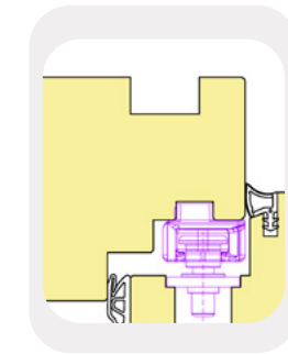
Option dormant avec rainure à plac
