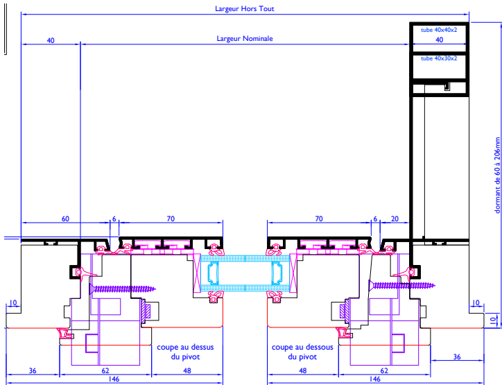
coupe horizontale
